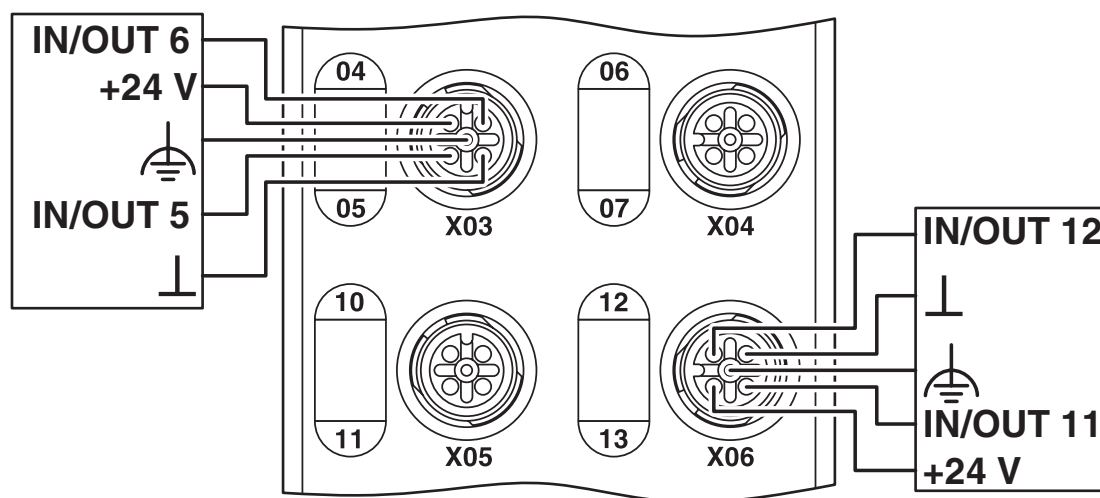
Disegno collegamento
