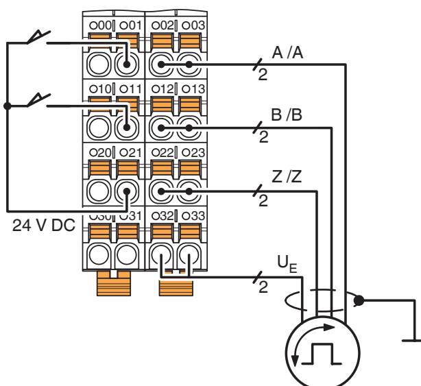
Disegno collegamento
