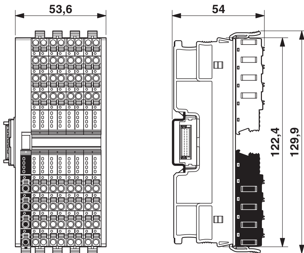
Disegno quotato
