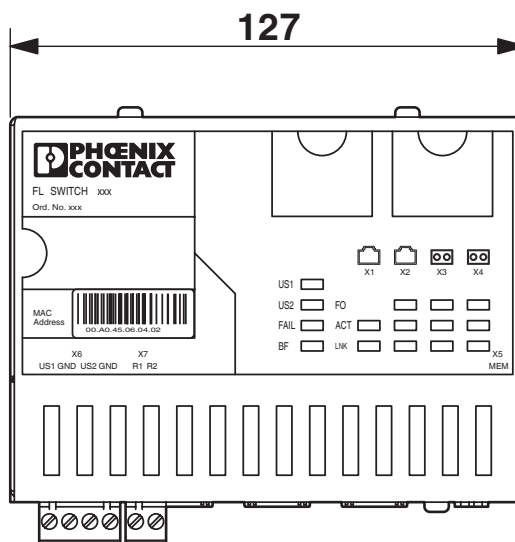
Disegno quotato
