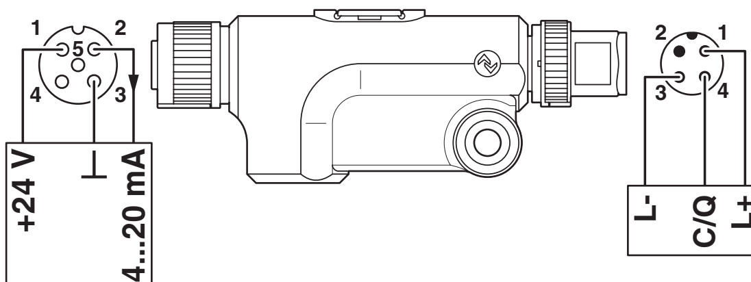
Disegno collegamento
