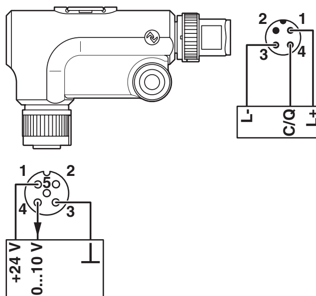
Disegno collegamento
