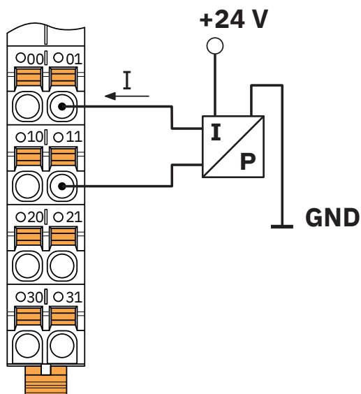
Disegno collegamento
