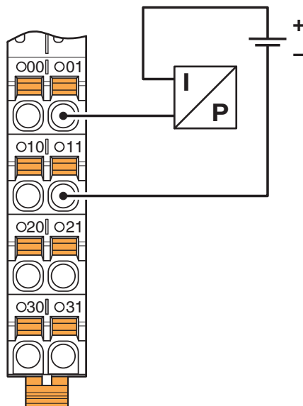
Disegno collegamento
