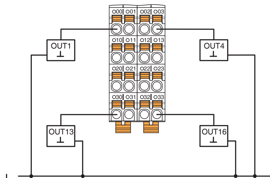
Disegno collegamento
