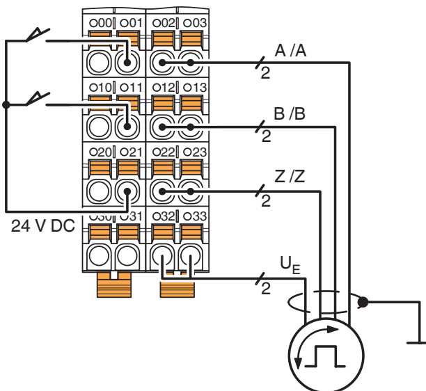
Disegno collegamento
