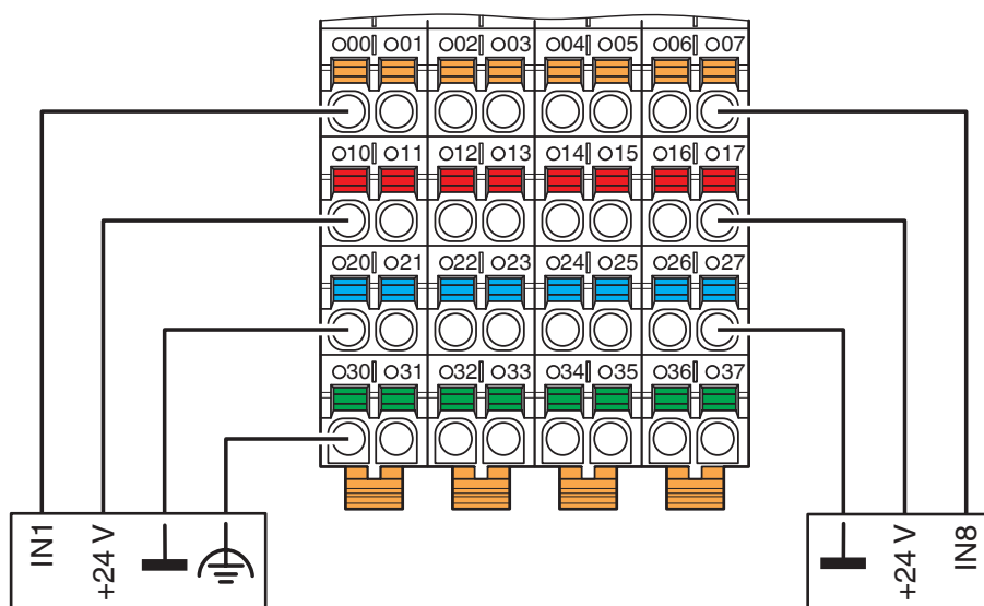
Disegno collegamento
