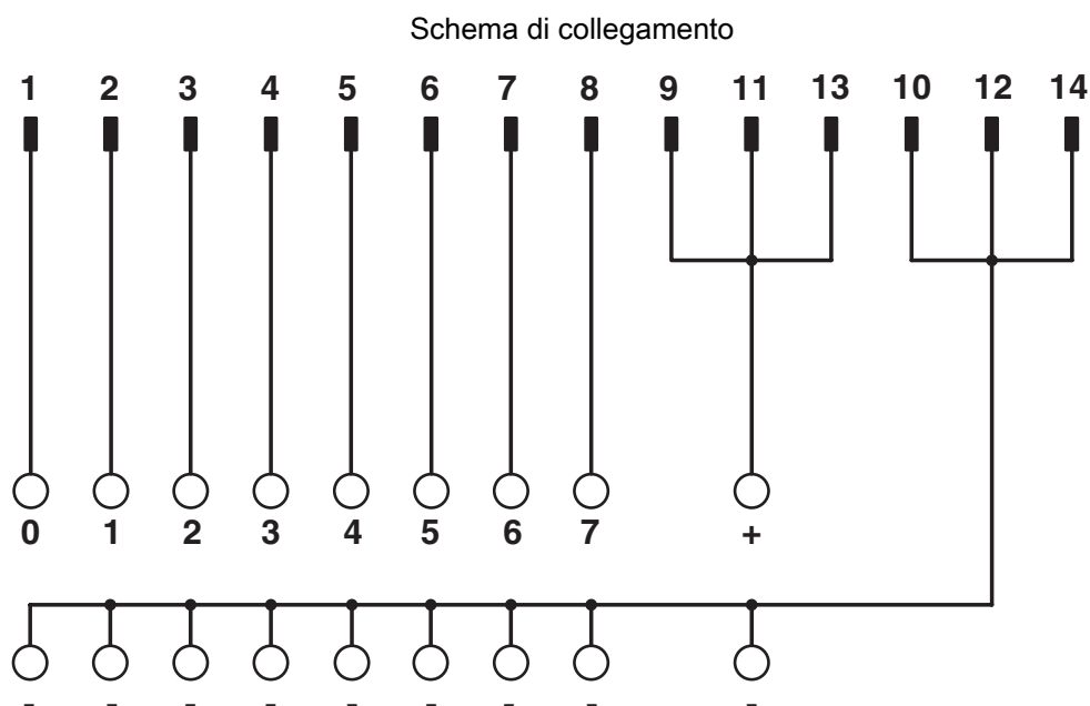
Schema di collegamento VIP-2/.../FLK14/8M/PLC
