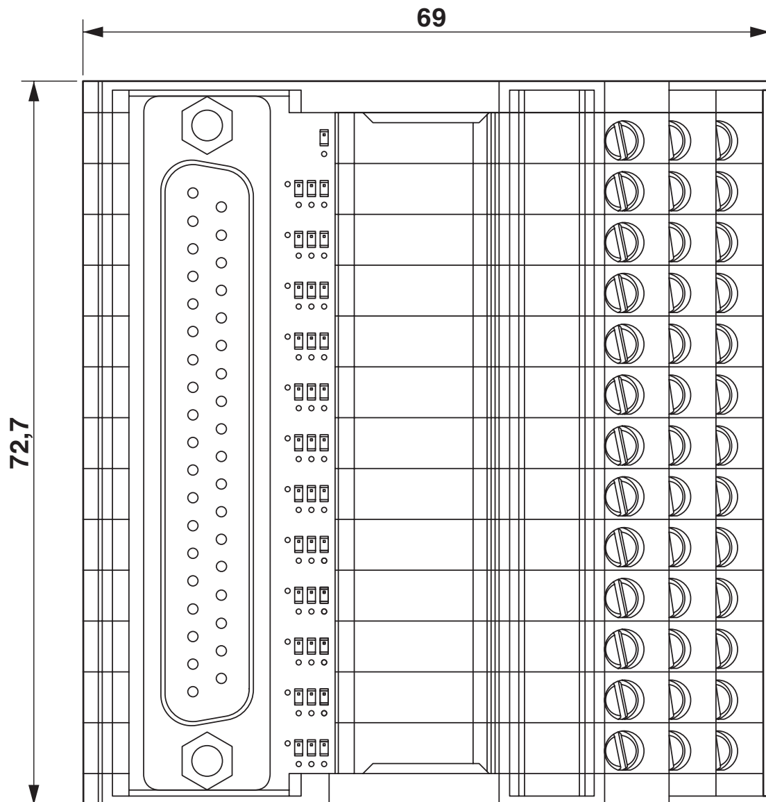
Disegno quotato
