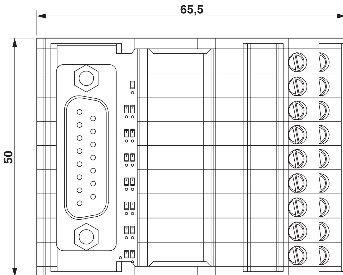
Disegno quotato
