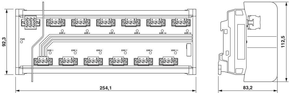
Disegno quotato
