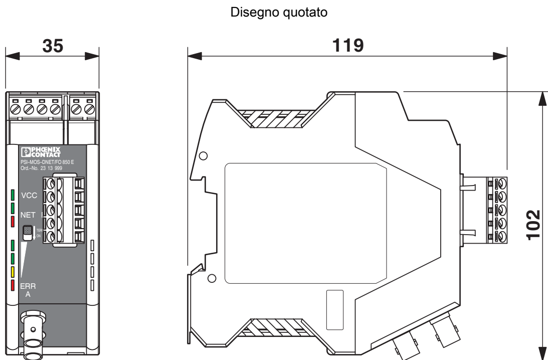
Dimensioni della custodia
