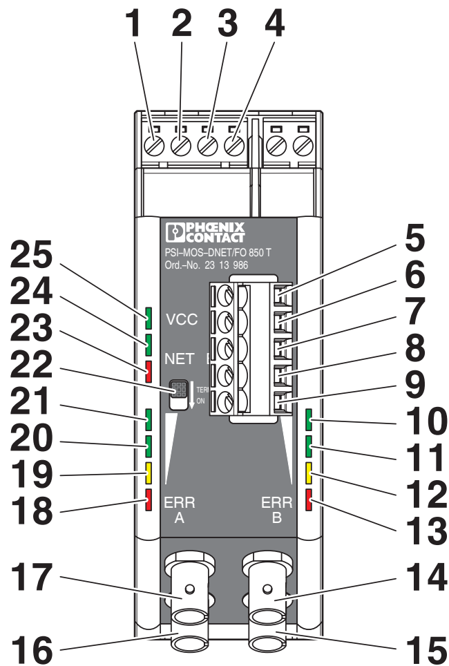
Disegno schema
