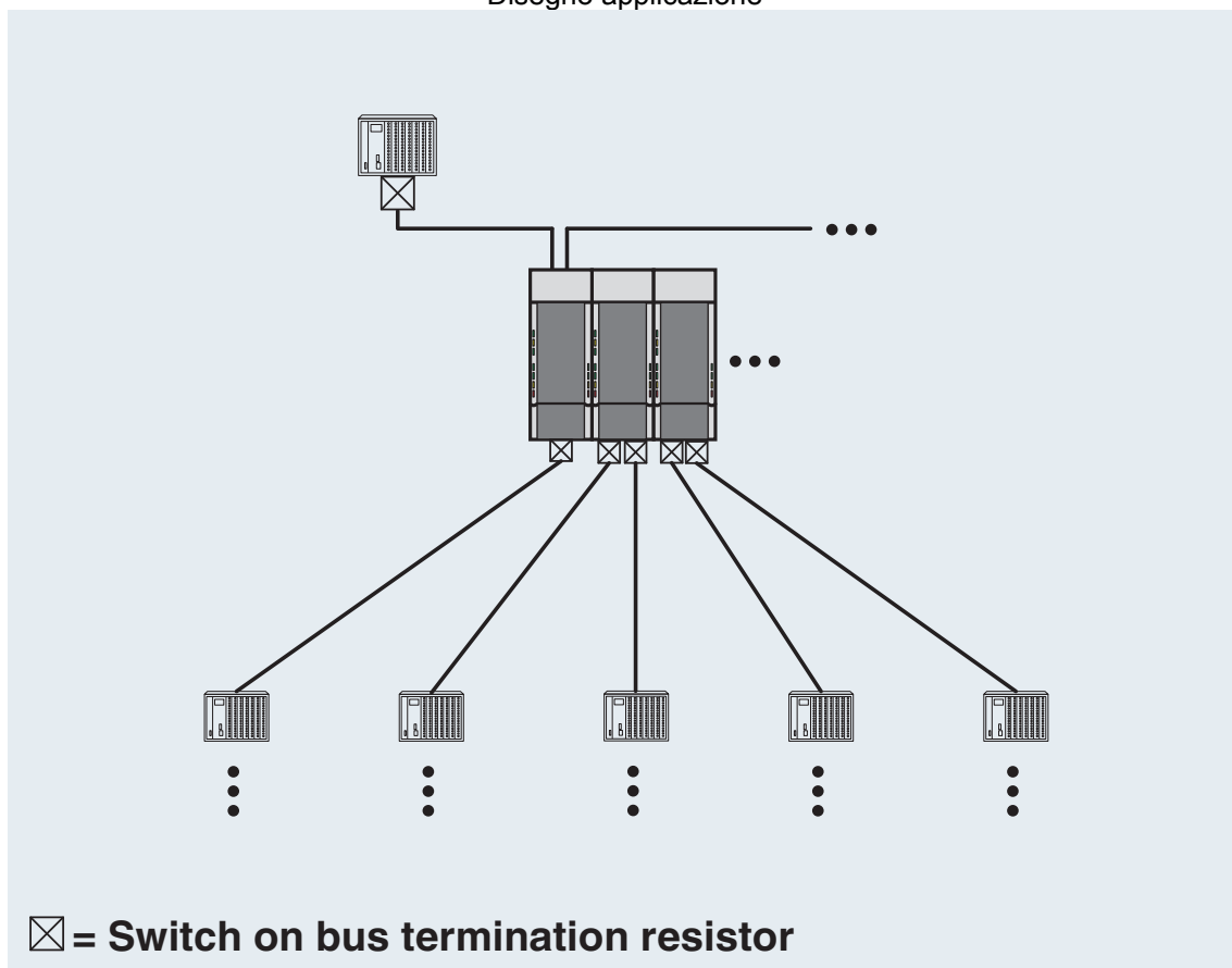
Disegno applicazione
