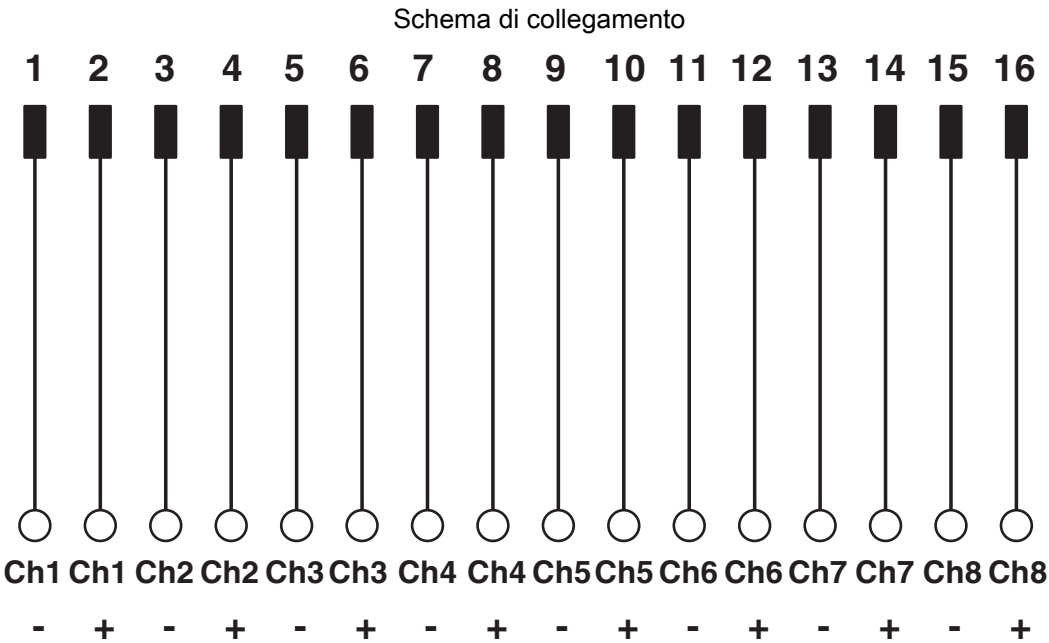
Schema di collegamento FLKM 16/DV
