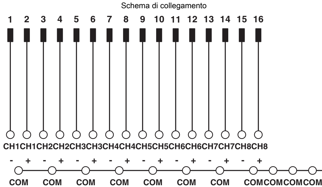
Schema di collegamento FLKM 16/AI/DV
