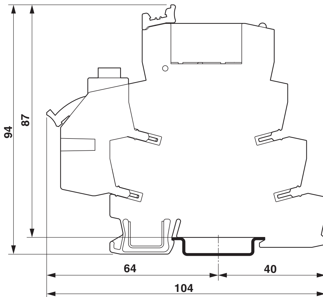
Disegno quotato
