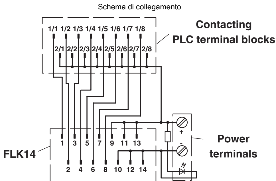
Schema di collegamento PLC-V8/FLK14/IN
