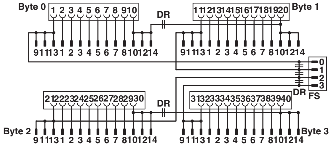
Schema di collegamento FLKM 50/4-FLK14/PA-S300
