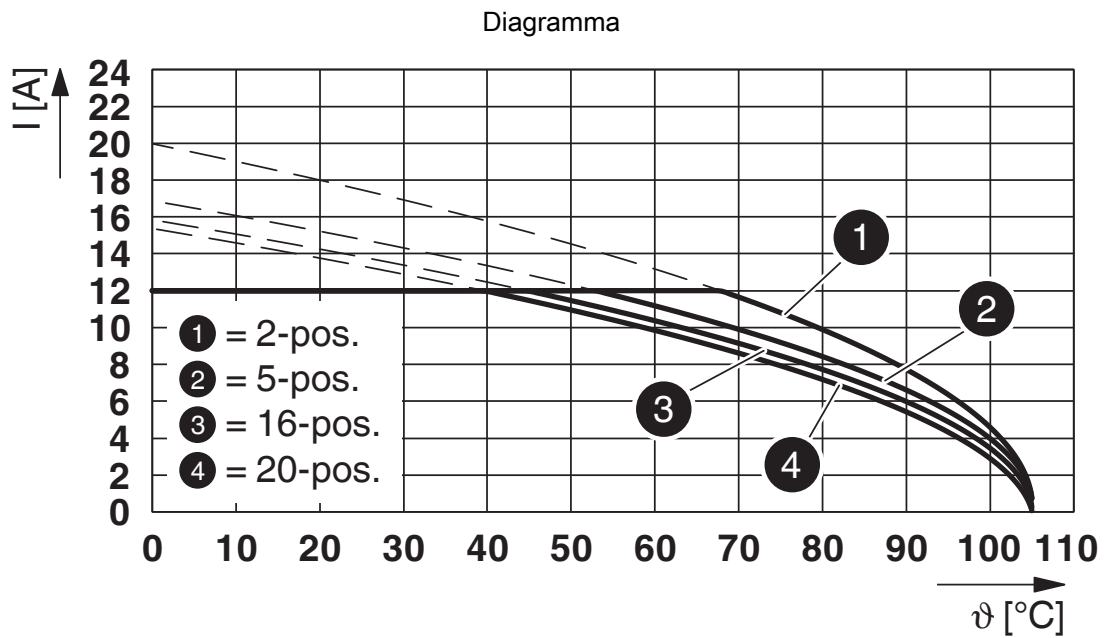
Tipo: FKCT 2,5/...-ST-5,08 con MSTBVA 2,5/...-G-5,08
