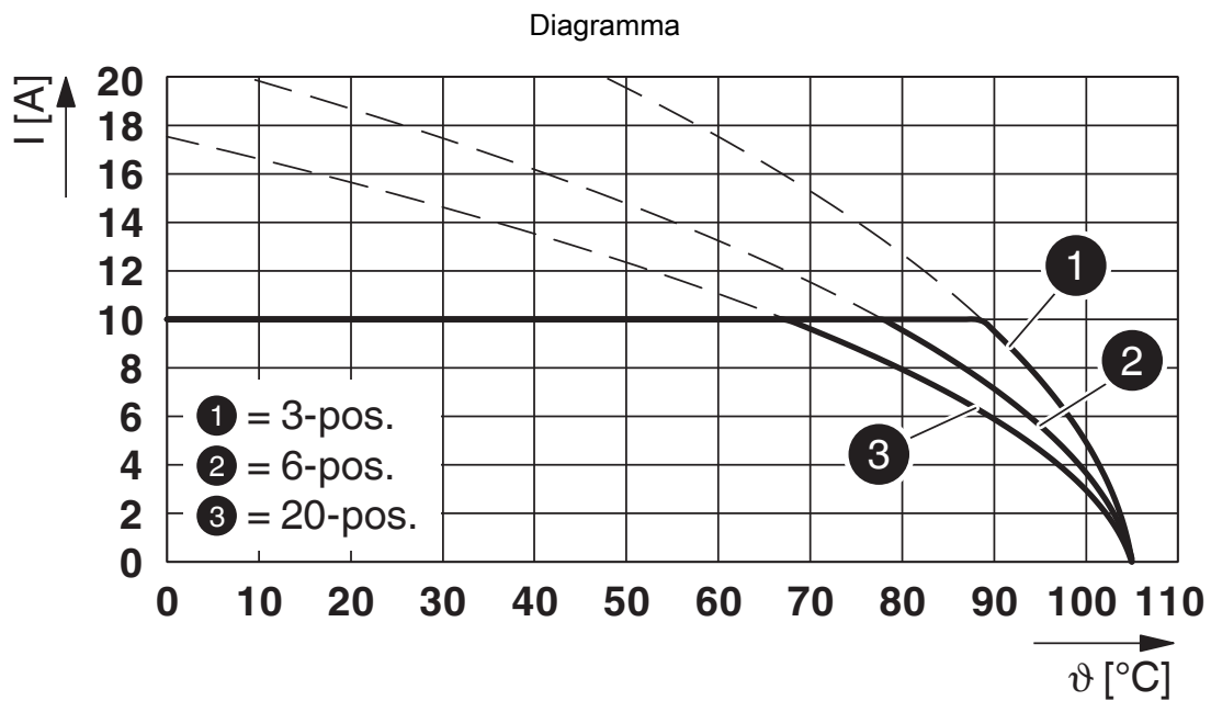
Tipo: FKCT 2,5/...-ST-5,08 con MDSTBV 2,5/...-G1-5,08
