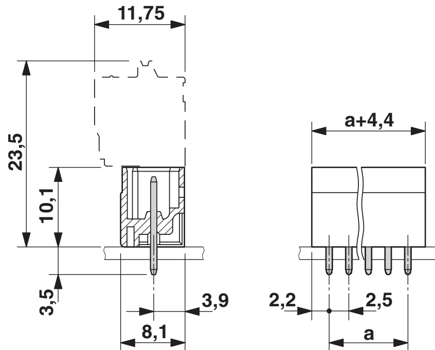
Disegno quotato
