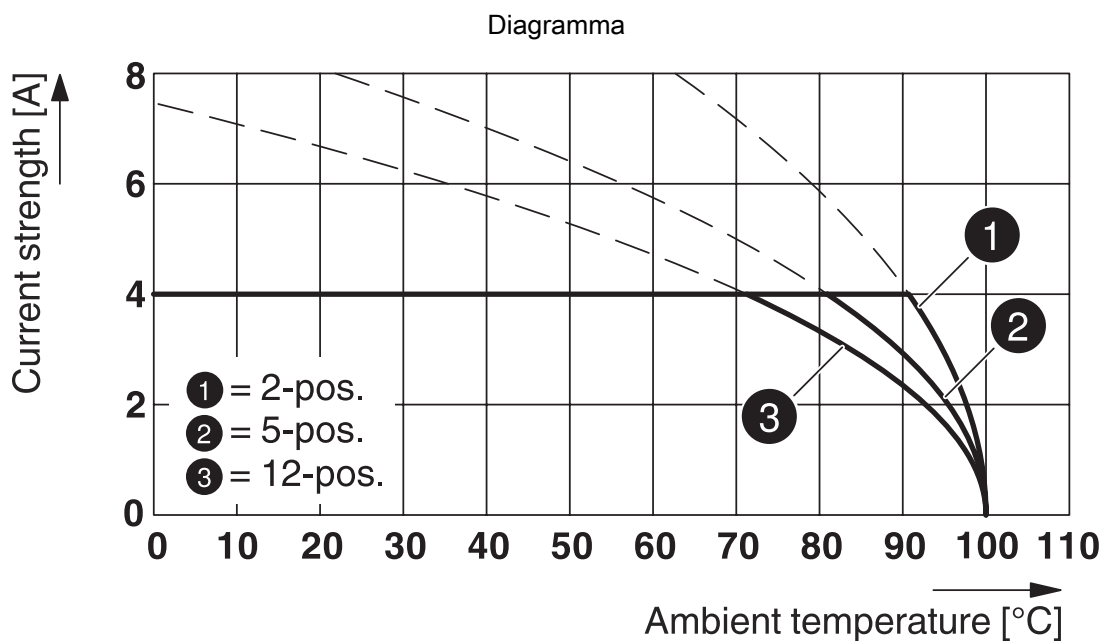
Tipo: FK-MC 0,5/...-ST-2,5 con MCD 0,5/...-G1-2,5 HT BK
