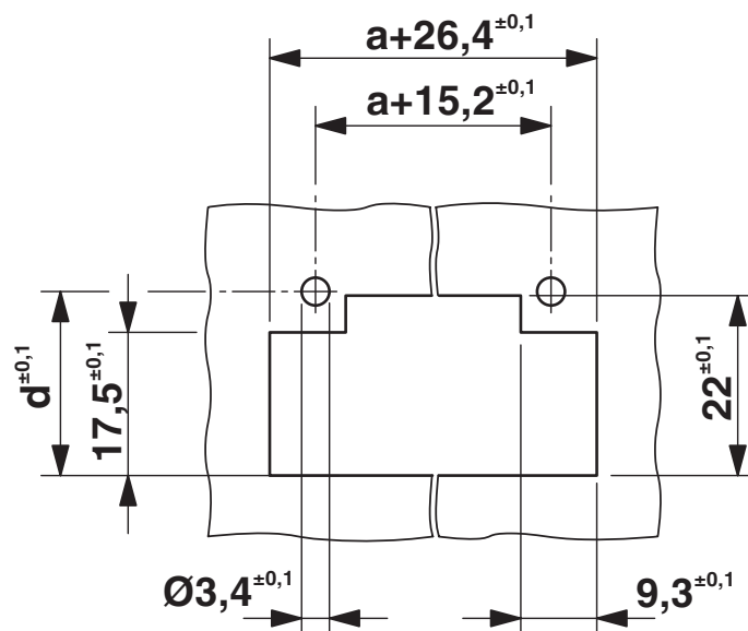
Disegno quotato
