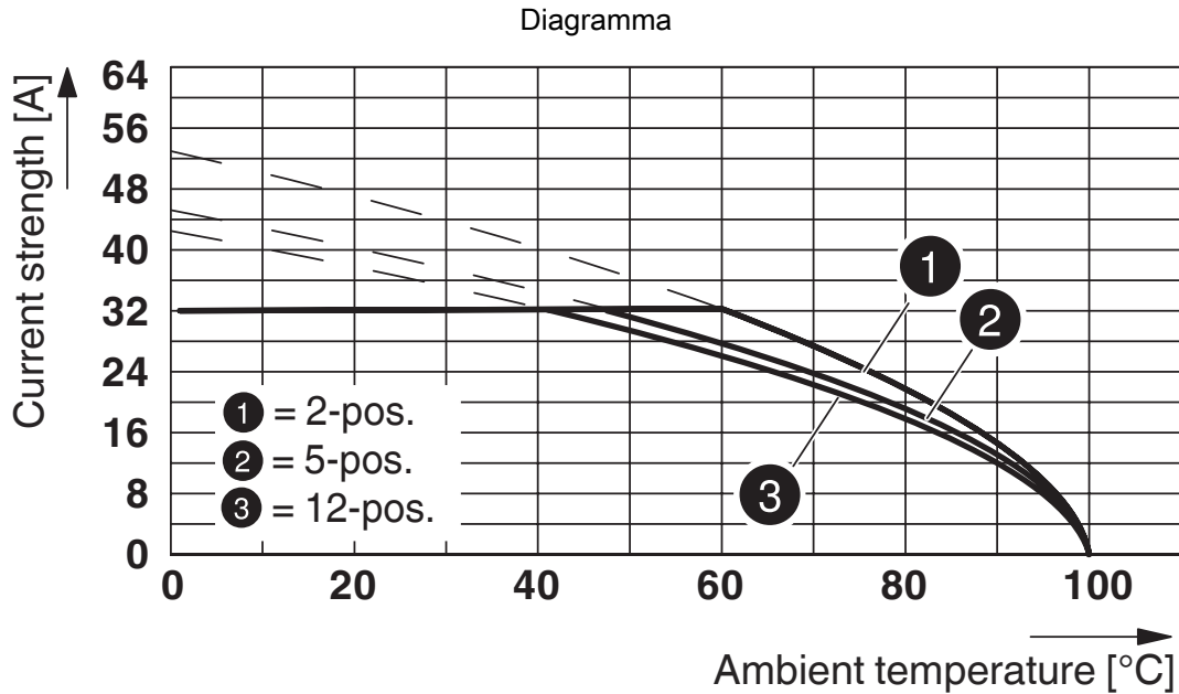
Tipo: PC 5/...-ST1-7,62 con PC 4/...-G-7,62 Sezione del conduttore: 6 mm 2
