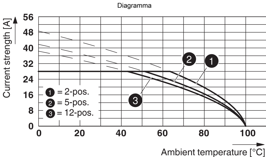
Tipo: PC 5/...-ST1-7,62 con PC 4/...-G-7,62 Sezione del conduttore: 4 mm 2
