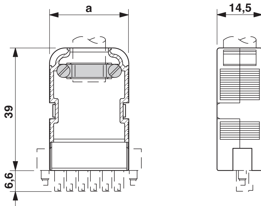
Disegno quotato
