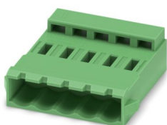
La figura illustra la versione a 10 poli
