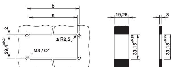
Disegno quotato
