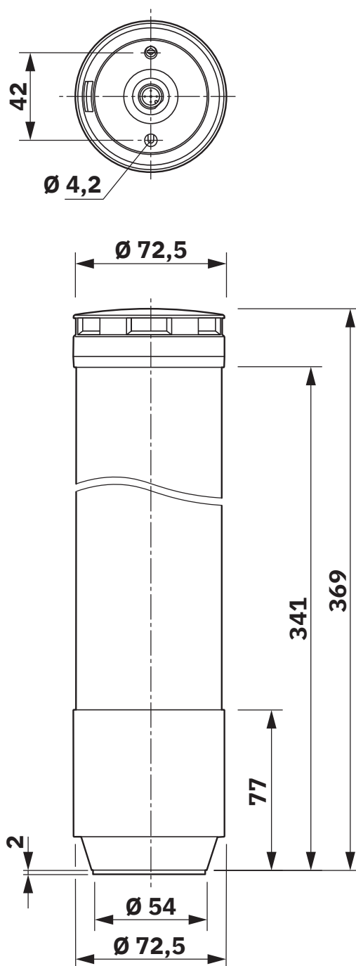
Disegno quotato
