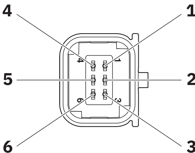
Disegno collegamento
