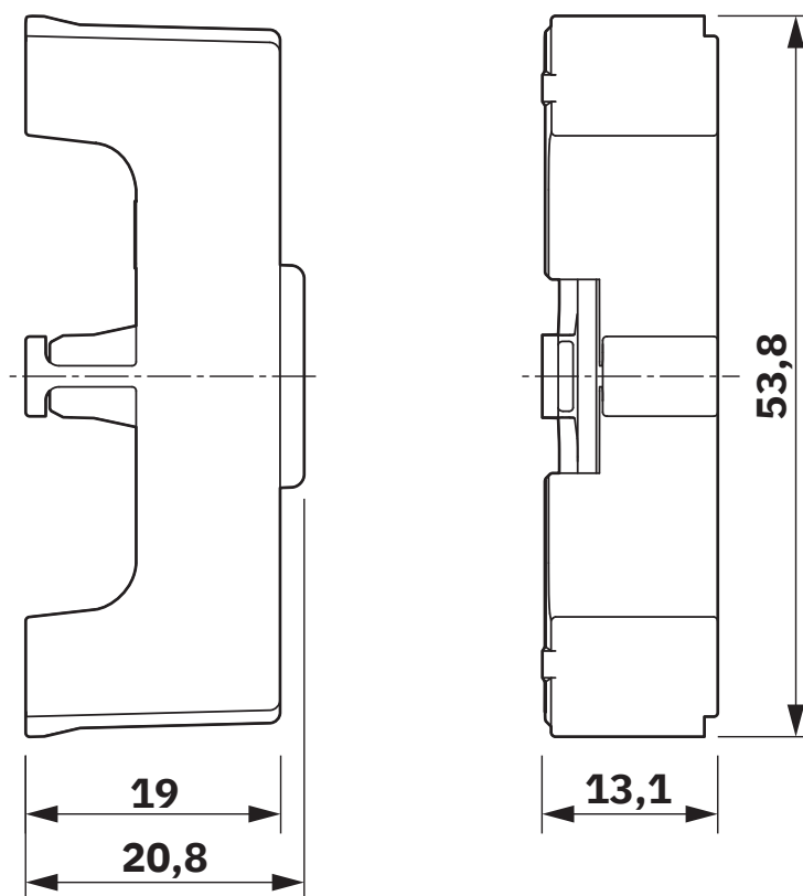
Disegno quotato
