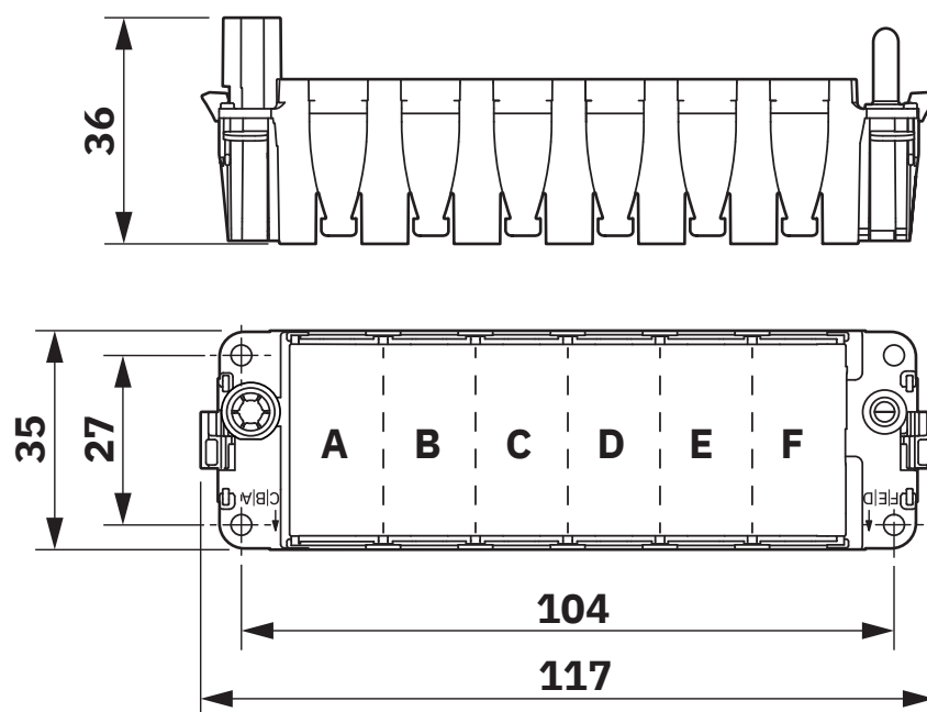
Disegno quotato
