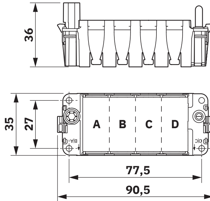
Disegno quotato
