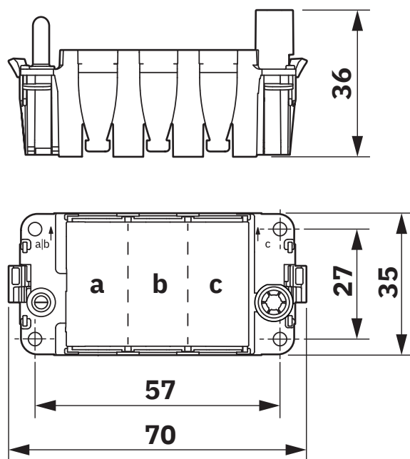
Disegno quotato
