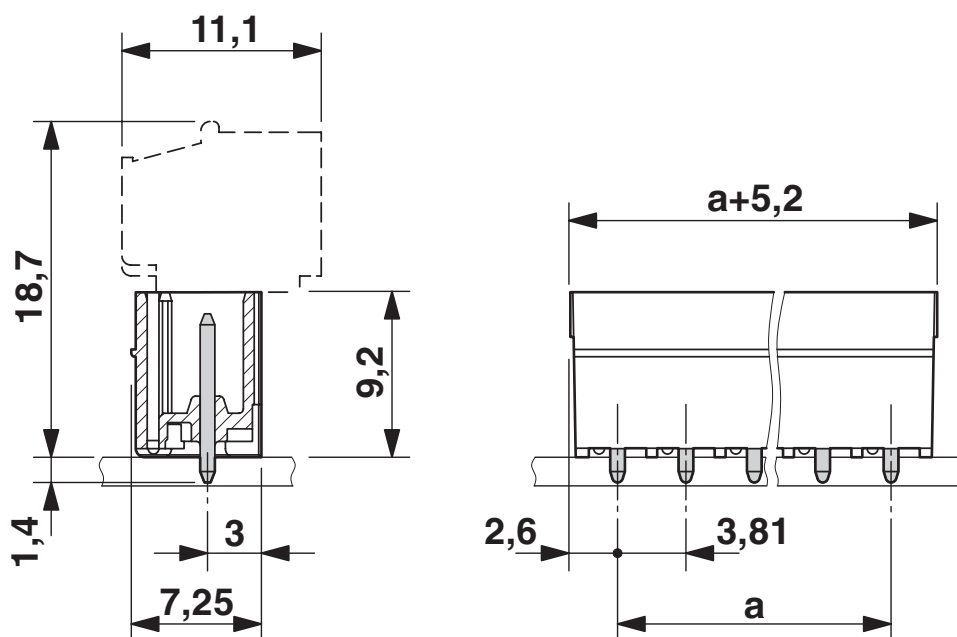
Disegno quotato
