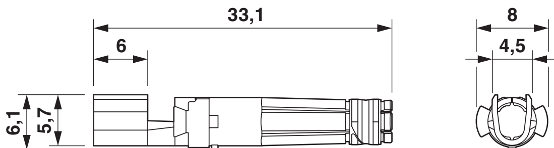
Disegno quotato
