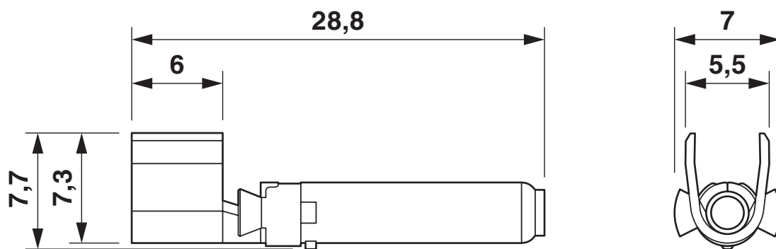
Disegno quotato
