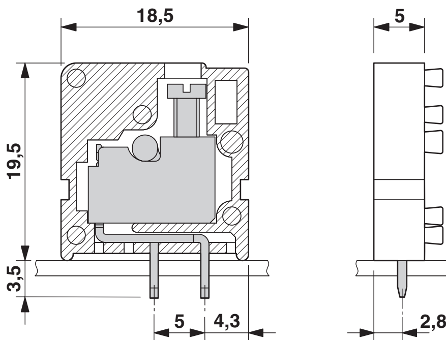
Disegno quotato
