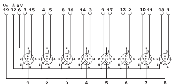
Schema di collegamento
