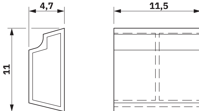
Disegno quotato
