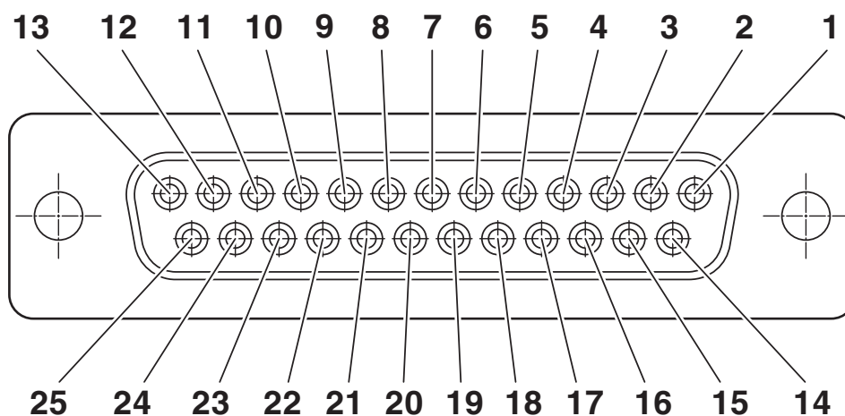
Disegno schema
