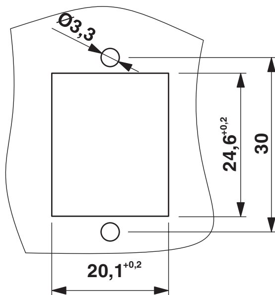
Disegno quotato
