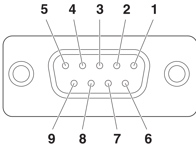
Disegno schema
