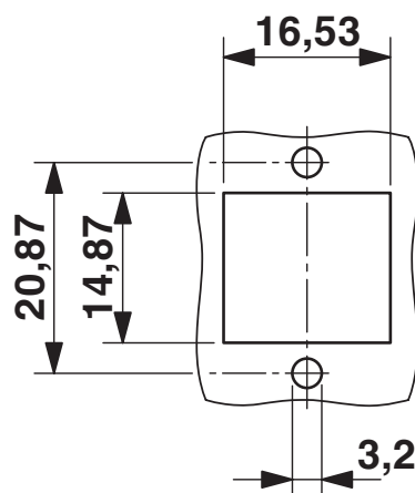
Disegno quotato
