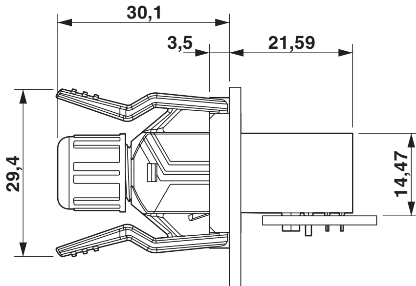
Disegno quotato
