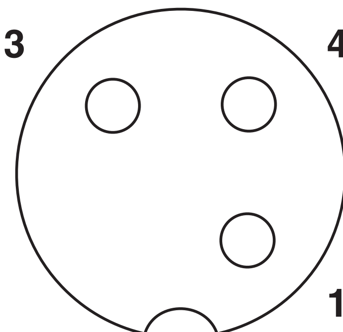
Disegno schema
