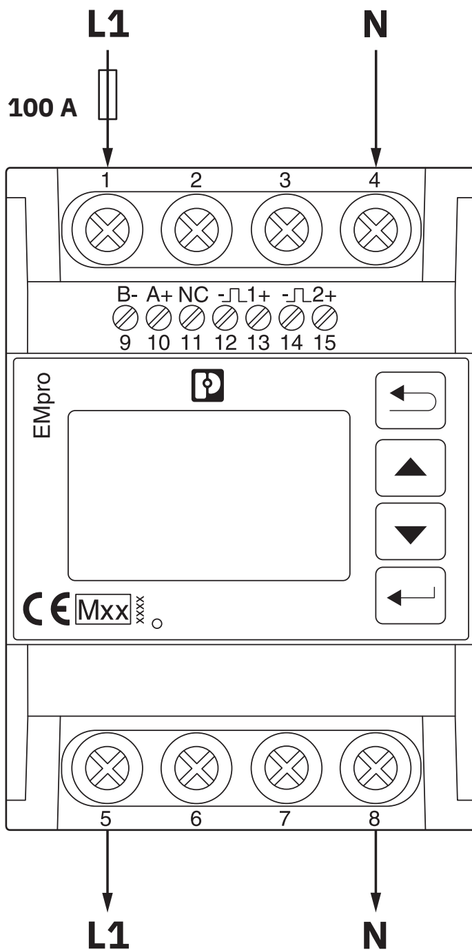
Disegno collegamento
