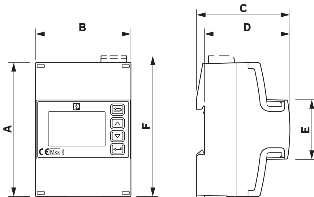
Disegno quotato
