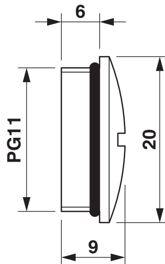
Disegno quotato
