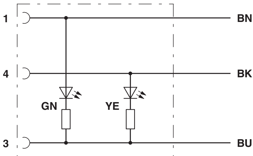
Equipaggiamento dei contatti dei connettori femmina M8 con 2 LED
