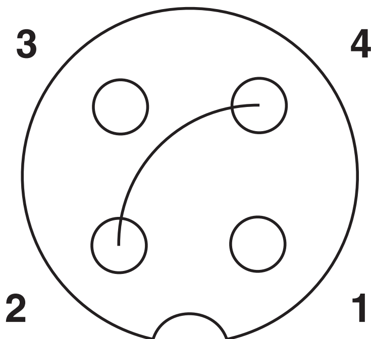
Disegno schema
